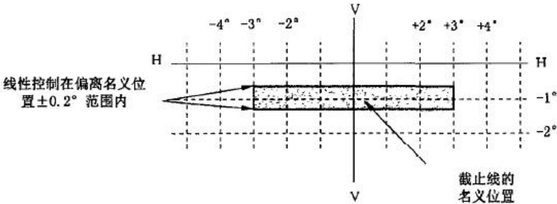
图 D.1 明暗截止线的位置和形状
