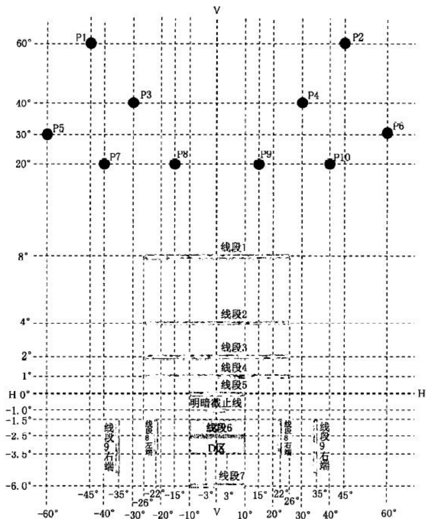
图 2 F3 级前雾灯配光屏幕
