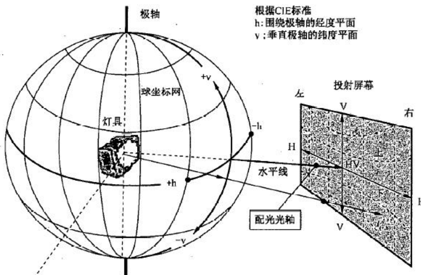
图 3 带极轴的球角度坐标测量网格
