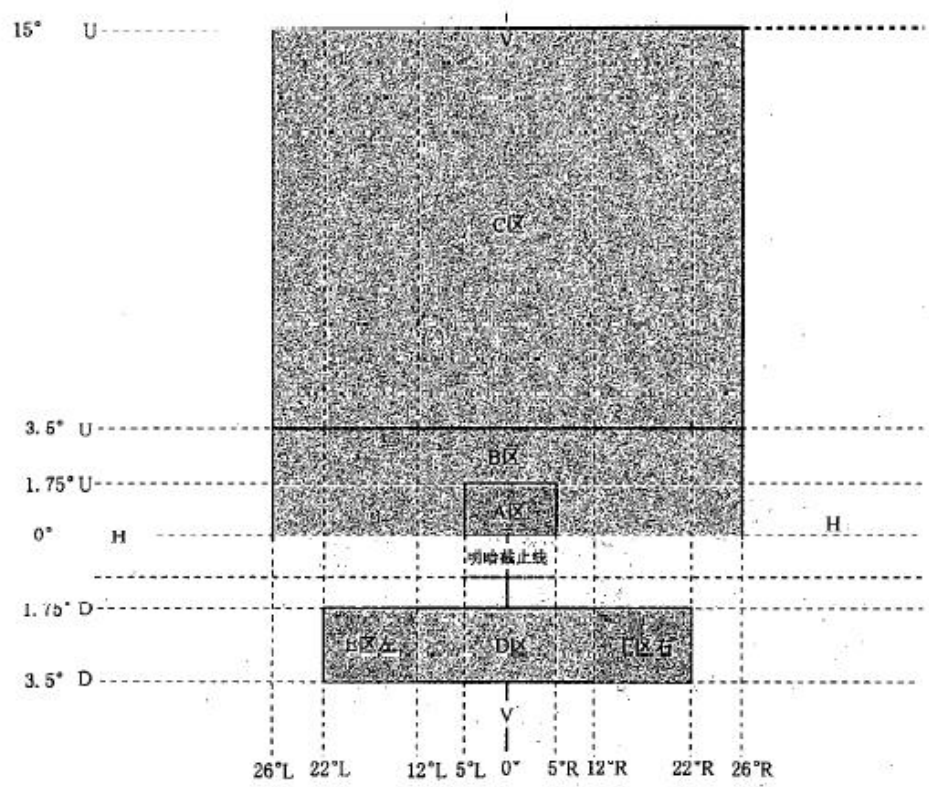
图 1 B 级前雾灯配光屏幕
